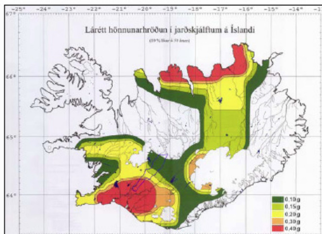
Mynd 22 Skipting Íslands í hönnunarhröðunarsvæði miðað við 500 ára meðalendurkomutíma. Heimild: Staðlaráð Íslands, Íslenskur staðall.
