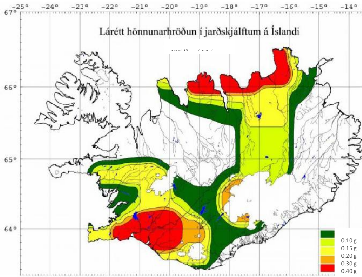
Mynd 13. Skipting Íslands í hönnunarhröðunarsvæði miðað við 50 ára meðalendurkomutíma. Heimild: Staðlaráð Íslands, Íslenskur staðall.
